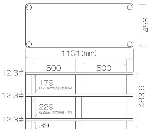
XW03G寸法図
