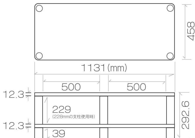
XW02G寸法図
