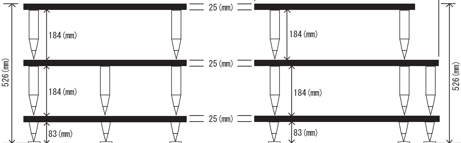
EXL2M1Cr 正面圖
