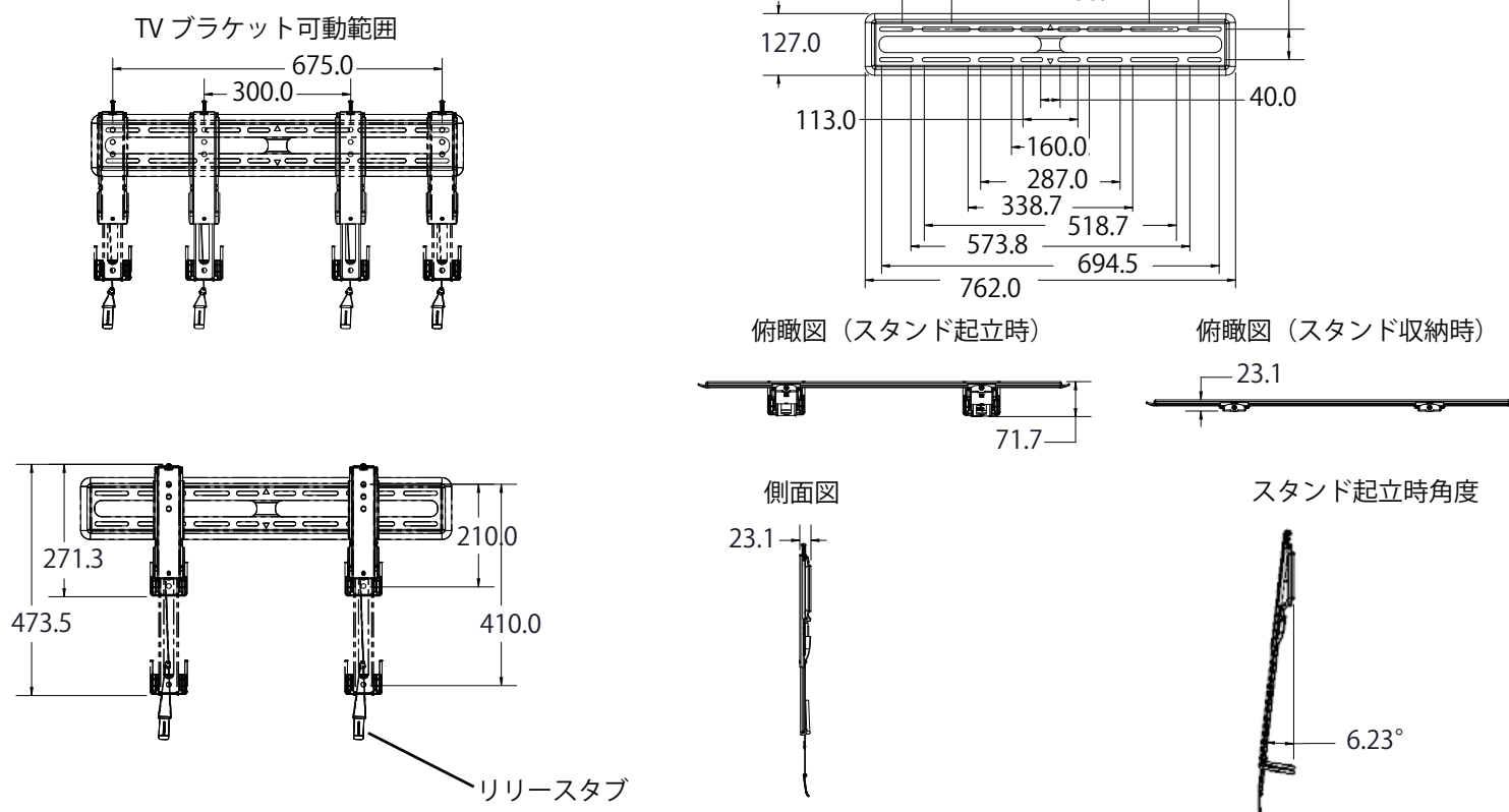
壁掛金具寸法図
