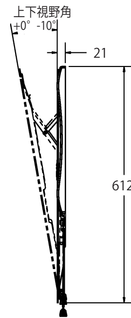
スタンドを収納した状態 (視野角 10°で使用状態)
