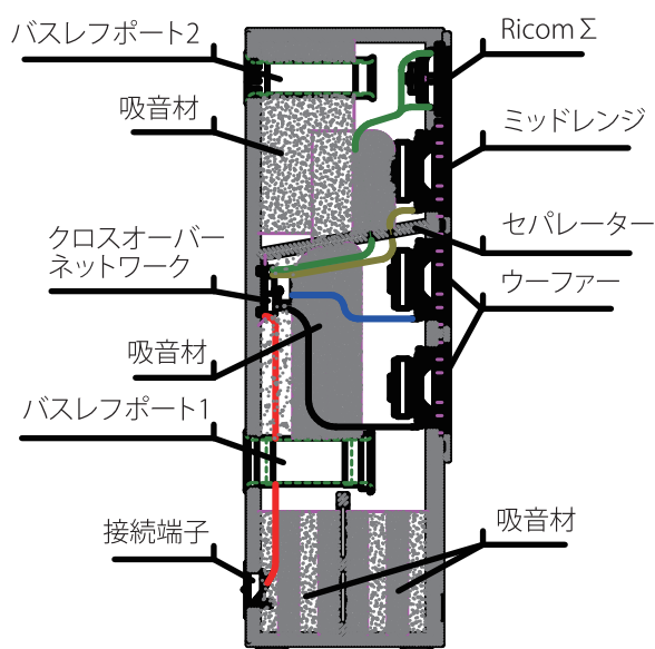
エンクロージャー内部構造 (SIGNUM70)
