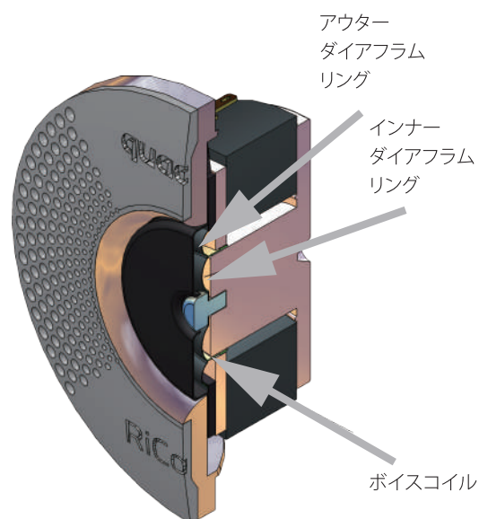
Ricom Σ トゥイーター内部構造
