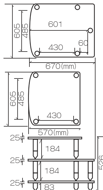
EXL2M1Cr寸法図
