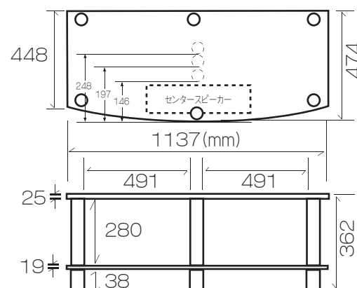
Ai02寸法図
