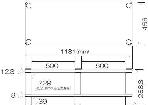
HXW02G寸法図 (製品重量 30.3 k g)
