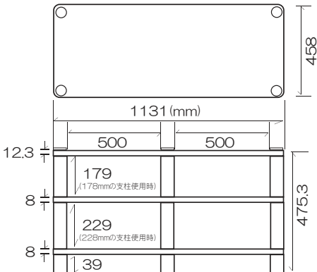
HXW03G寸法図 (製品重量 42.2 k g)
