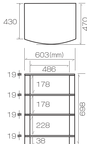
HFシリーズ寸法図
