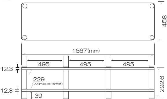
XWL03G寸法図 (製品重量 77.3 k g)
