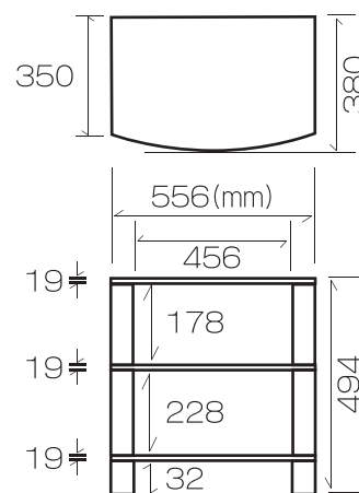
HSシリーズ寸法図
