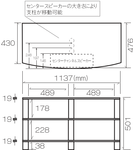
AV03シリーズ寸法図
