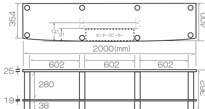
Ai222寸法図
