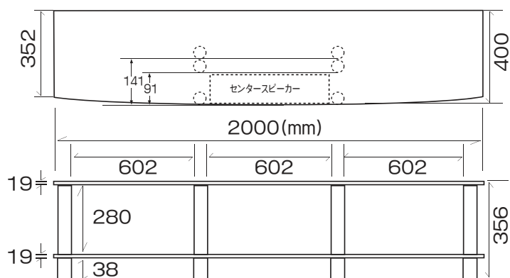
AV200寸法図
