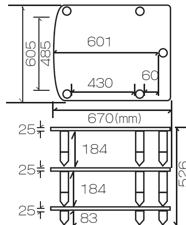
EXL3Cr寸法図
