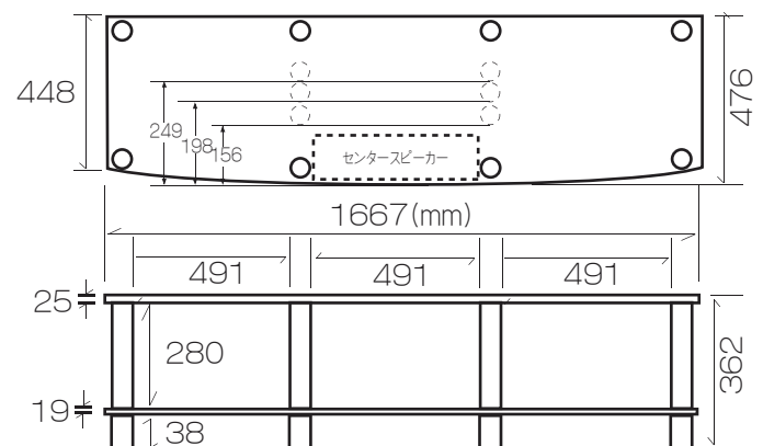
Ai22寸法図
