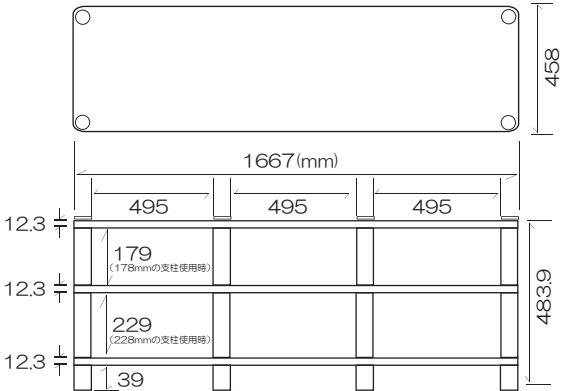
XWL03G寸法図 (製品重量 77.3 k g)
