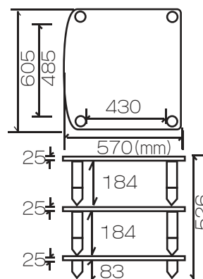
EXM3Cr寸法図
