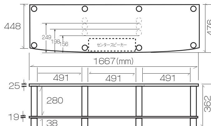
Ai22寸法図
