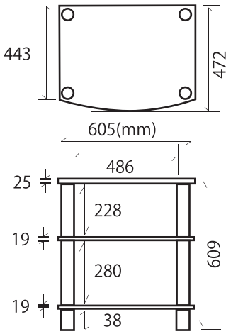
Hi03寸法図
