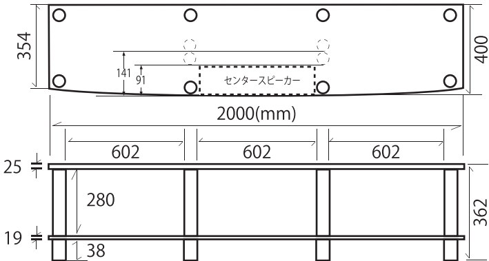
Ai222寸法図
