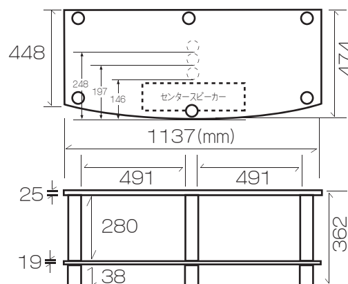
Ai02寸法図
